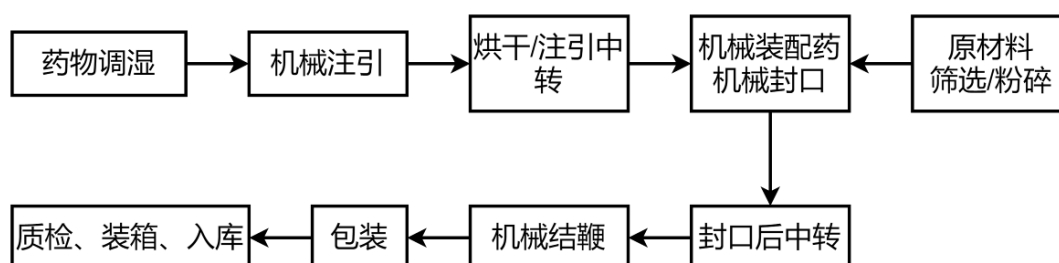
图 2-1：C 级爆竹类产品生产（注引）工艺流程
